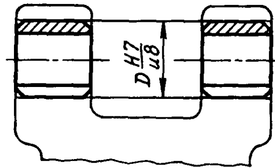
Рис. 11. Пример применения втулок без буртика
