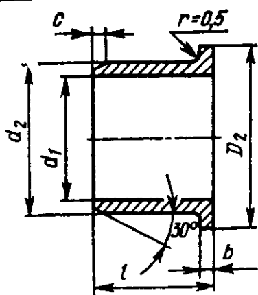
30б. Основные размеры, мм, втулок из термопластов
