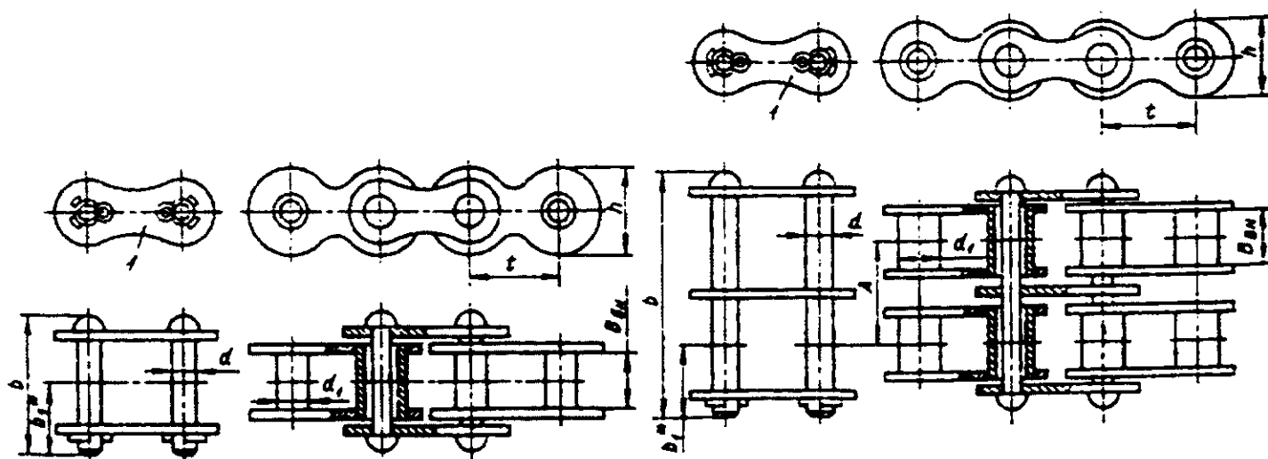
Однорядная типа ПВ
