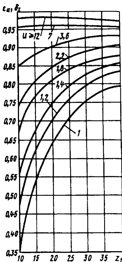
Рис. 58. График для определения значений \epsilon_{a1} \delta_I и \epsilon_{a2} \delta_{II} для косозубых передач без смещения при \beta < 15^\circ (на кривых показаны значения u )
