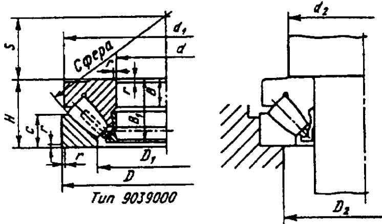
Размеры, мм
