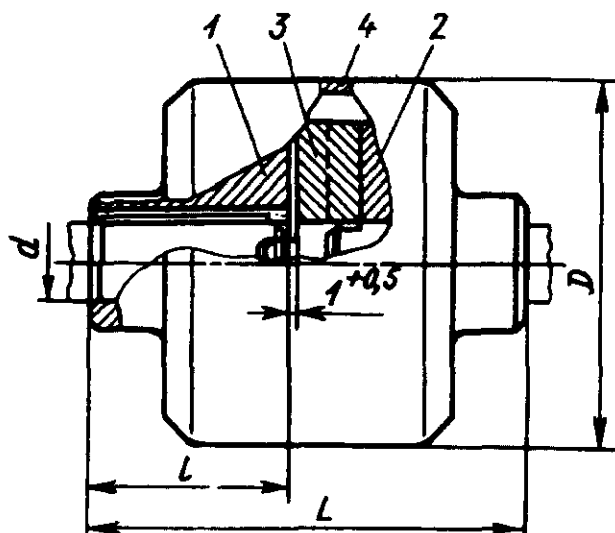
Исполнения 1 и 2
