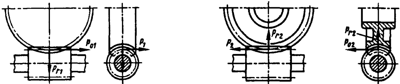
Силы, действующие на червяк
