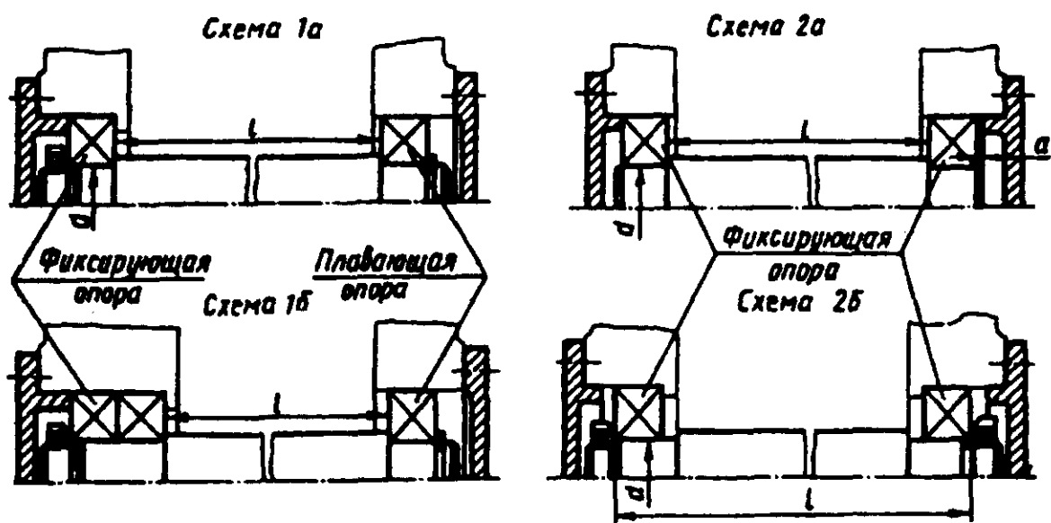
Рис. 24. Способы осевого фиксирования валов
