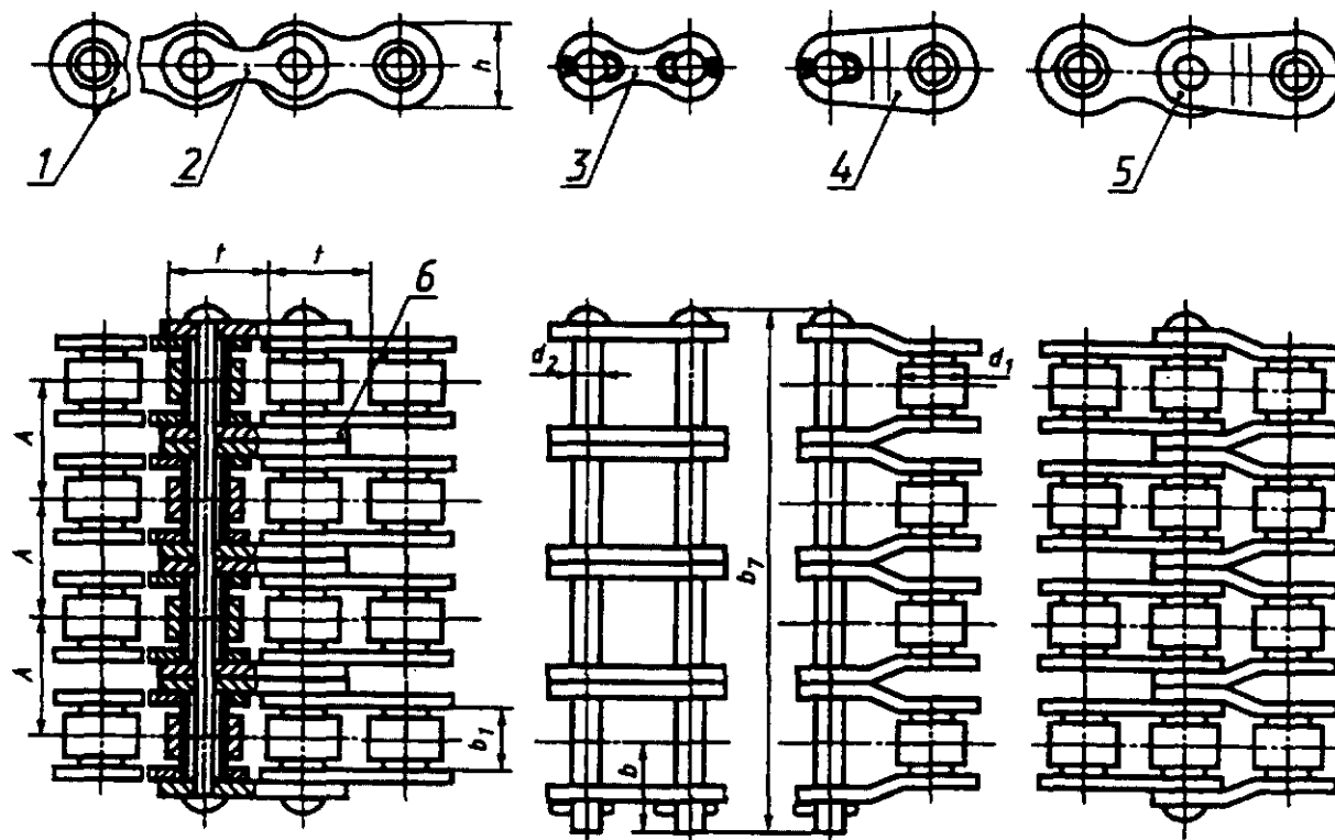
Цепи приводные роликовые четырехрядные типа 4ПР
