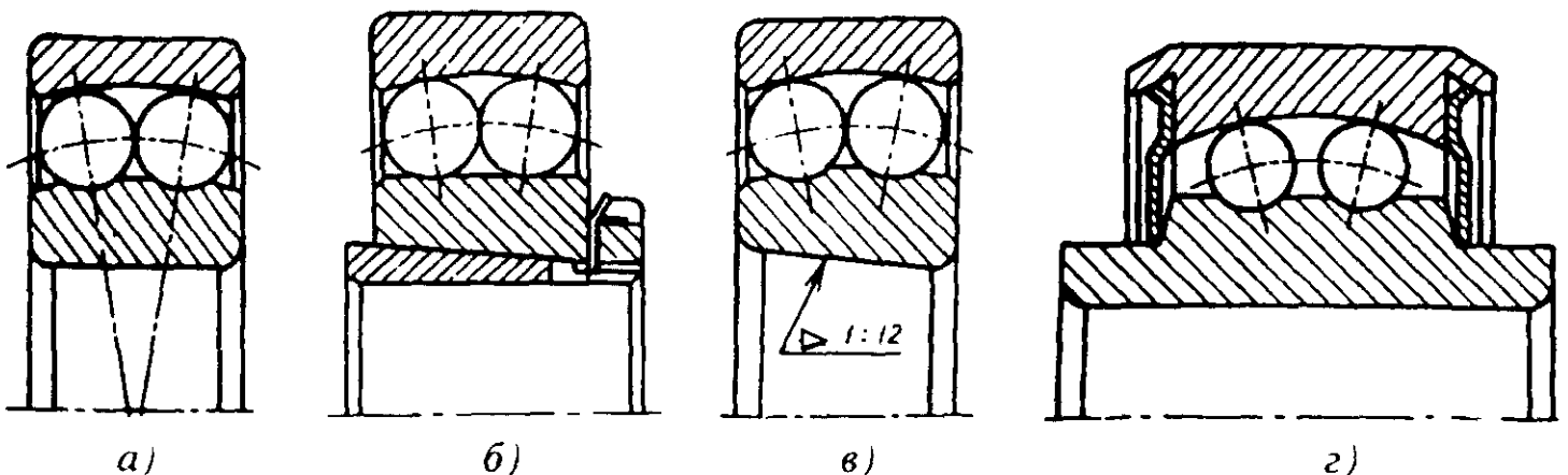
Рис. 14. Подшипники радиальные шариковые сферические исполнений:
