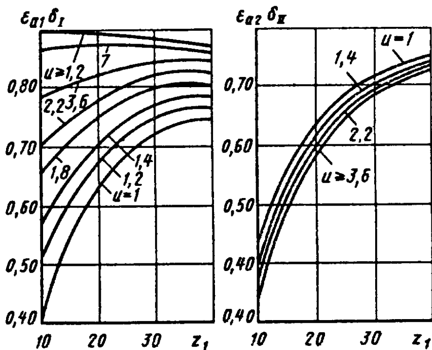
Рис. 59. График для определения значений \epsilon_{a1} \delta_I и \epsilon_{a2} \delta_{II} для косозубых передач без смещения при 15^\circ \leq \beta \leq 27^\circ
